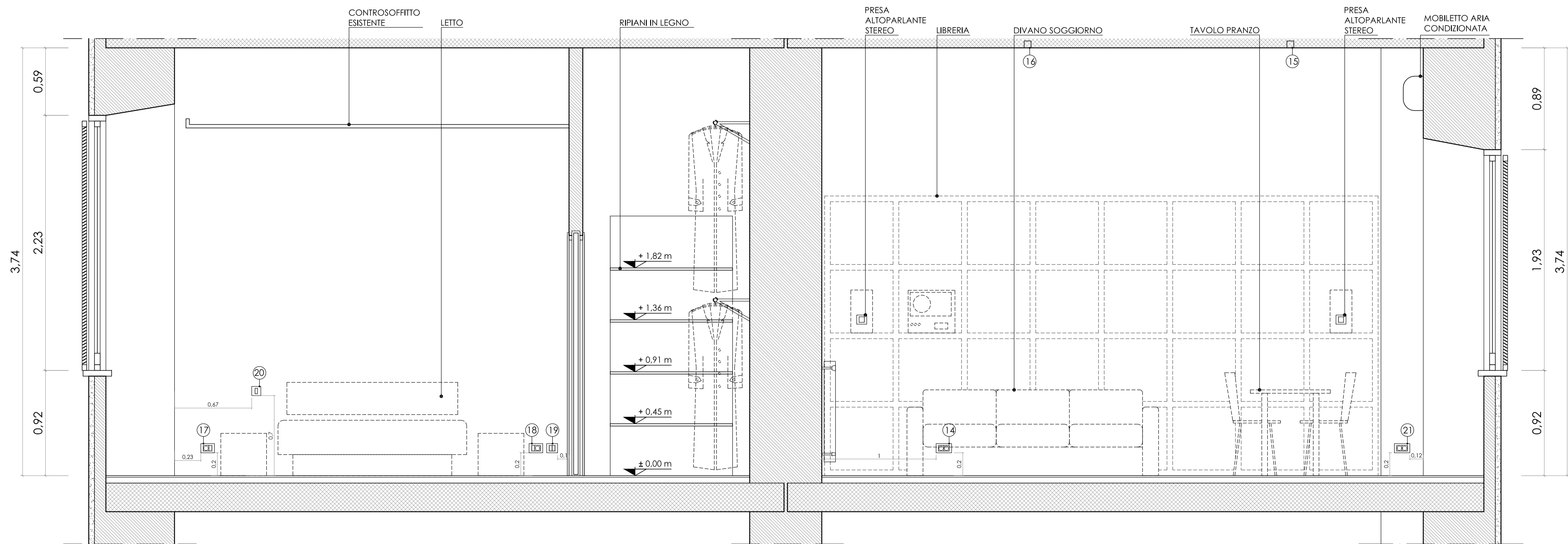
Sezione C-C' Rapp. 1/20
