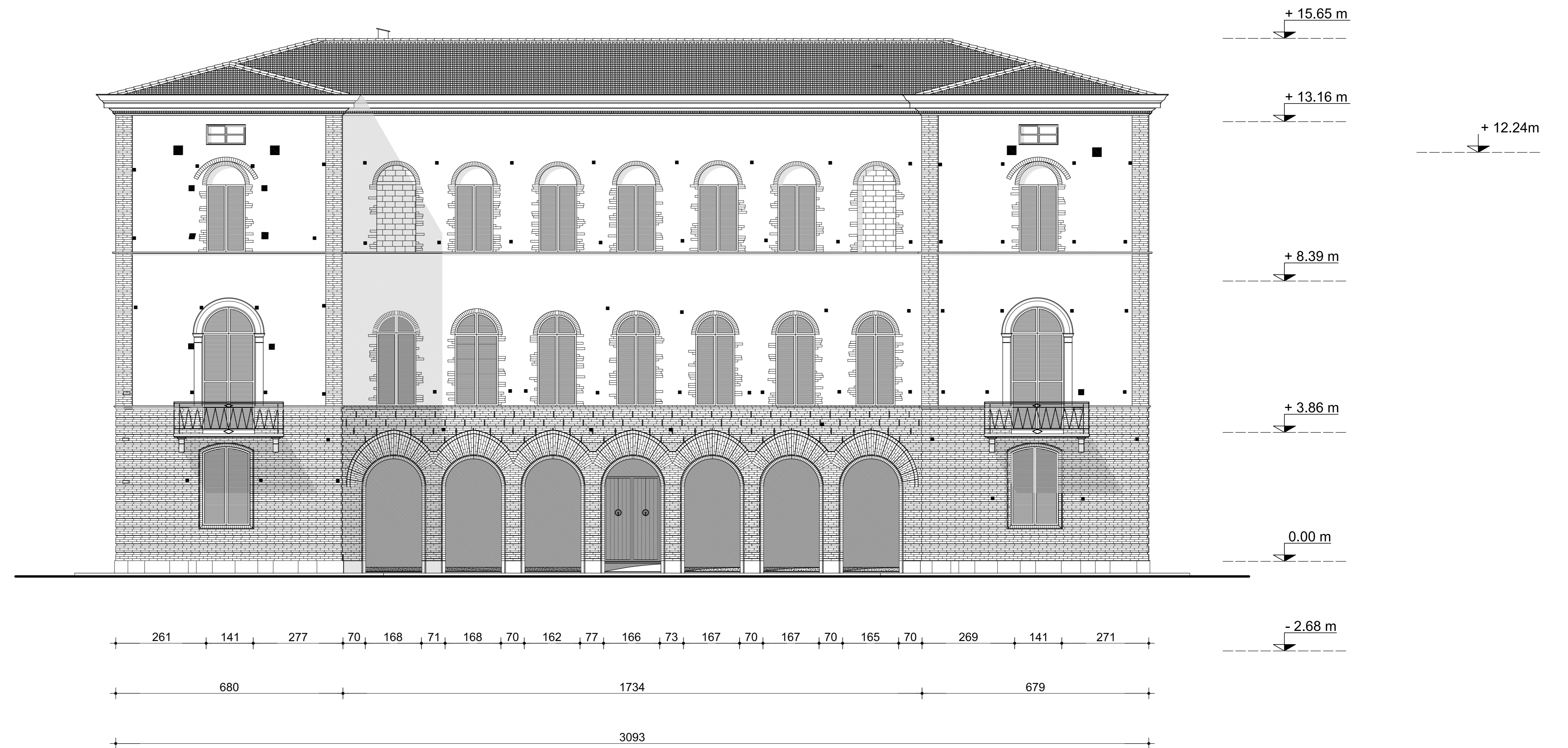
Prospetto SE
